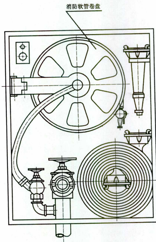
图 3 卷置式消火栓箱(配置消防软管卷盘)
