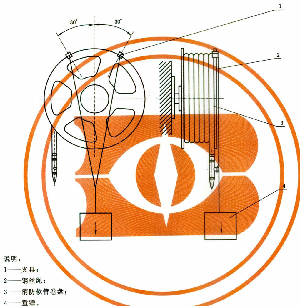
图 11 消防软管卷盘的负荷性能试验
