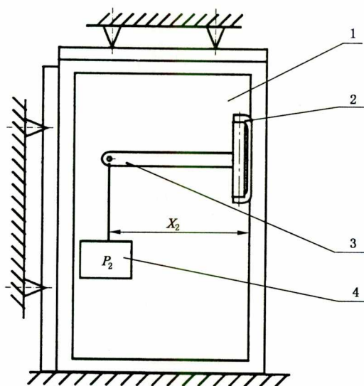
图 7 挂式消防栓箱的刚度试验
