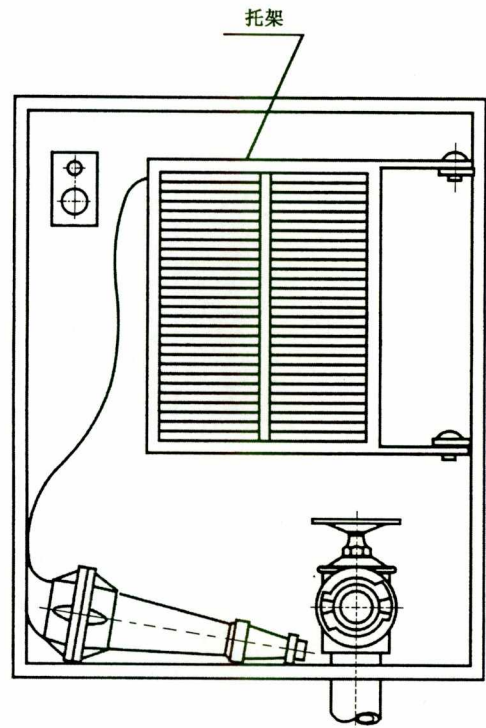
图 4 托架式消火栓箱
