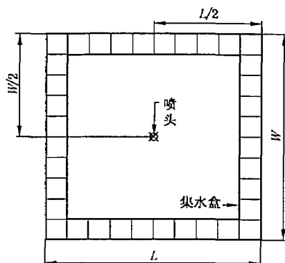
图 4 非边墙型家用喷头墙面布水试验布置图
